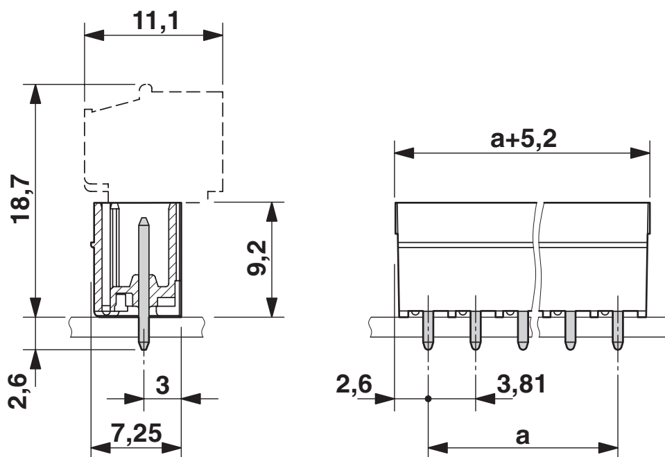
Maatschets
