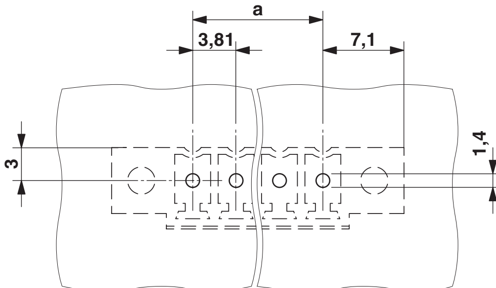
boorsjabloon/soldeerpadgeometrie
