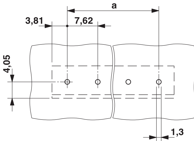
boorsjabloon/soldeerpadgeometrie
