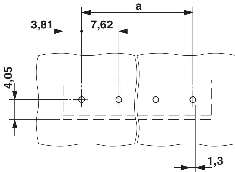
boorsjabloon/soldeerpadgeometrie
