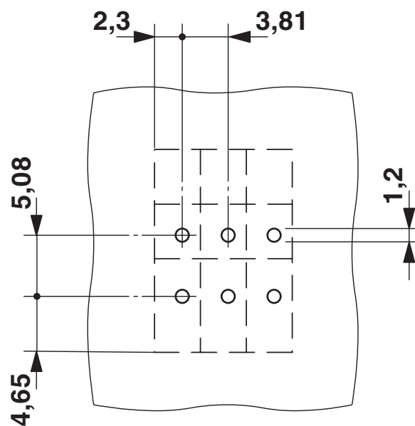
boorsjabloon/soldeerpadgeometrie
