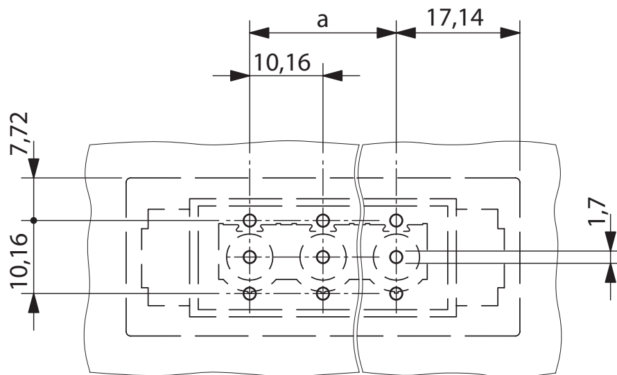
boorsjabloon/soldeerpadgeometrie
