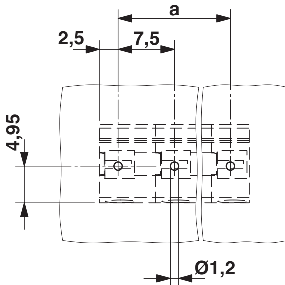
boorsjabloon/soldeerpadgeometrie
