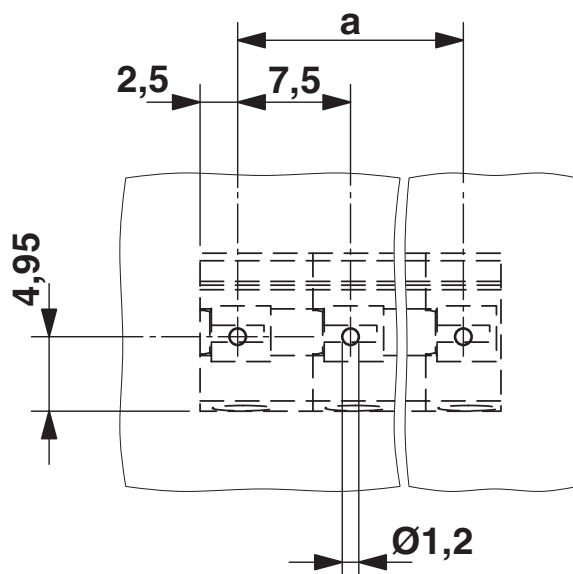
boorsjabloon/soldeerpadgeometrie
