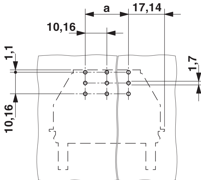
boorsjabloon/soldeerpadgeometrie
