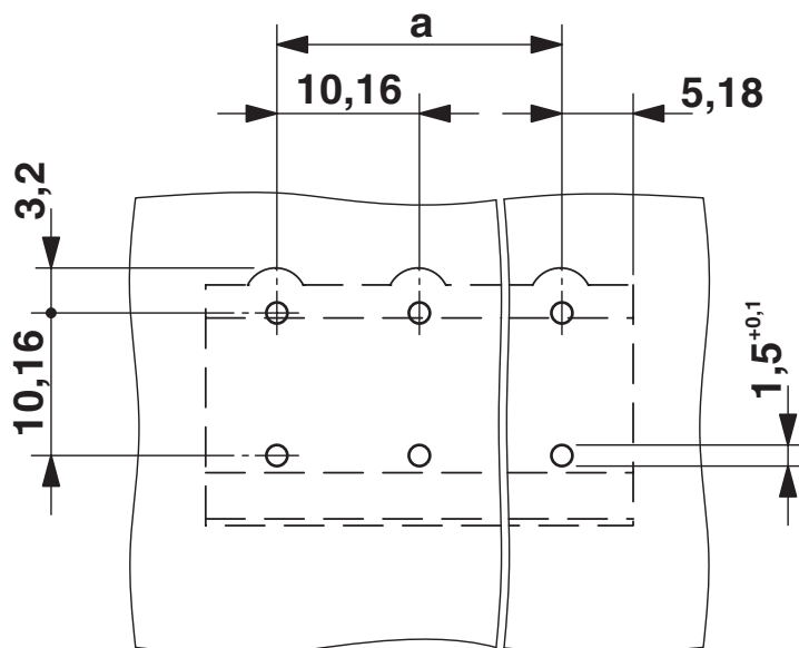
boorsjabloon/soldeerpadgeometrie
