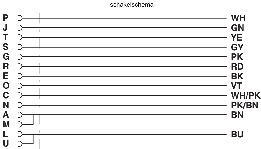
Contactbezetting van de M16-bus
