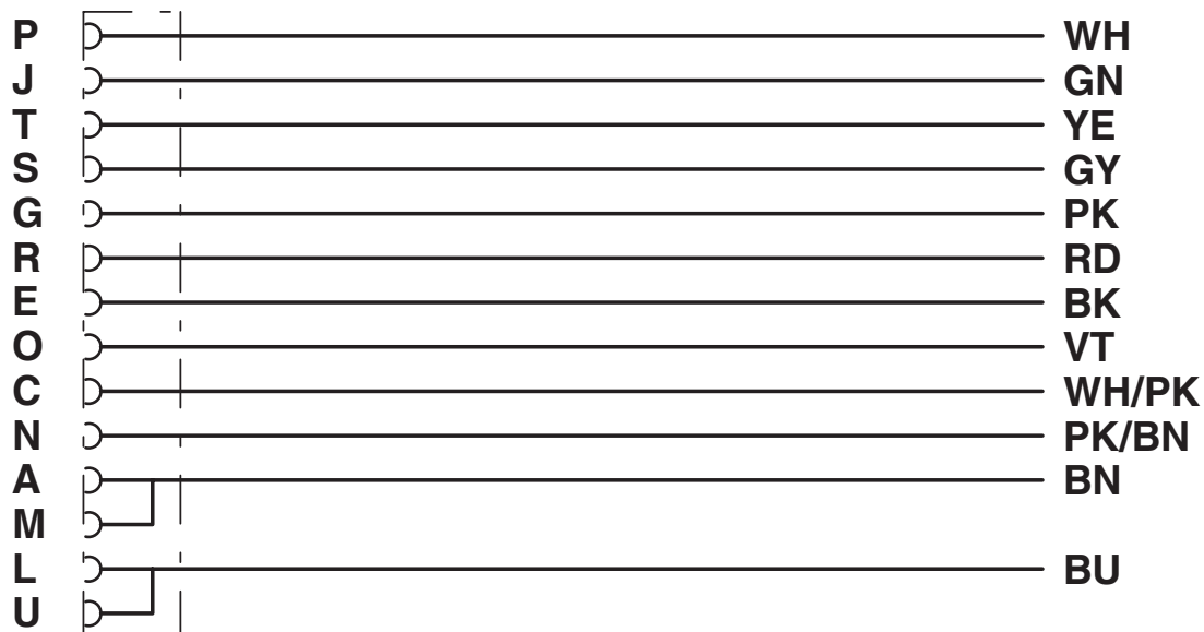
schakelschema
