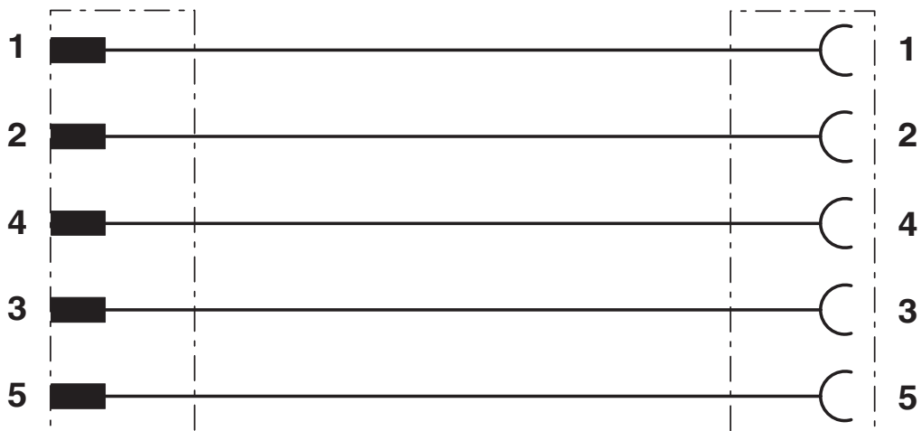
schakelschema
