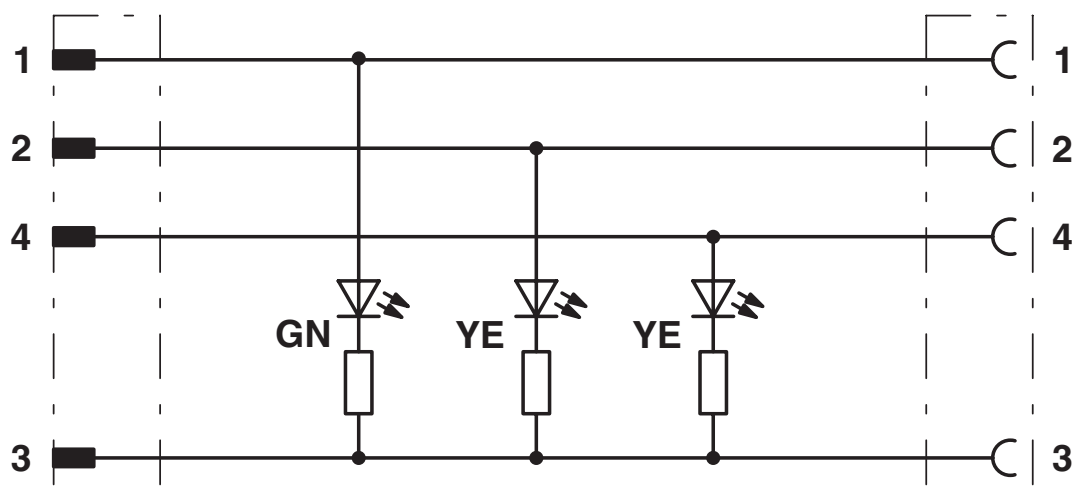
schakelschema
