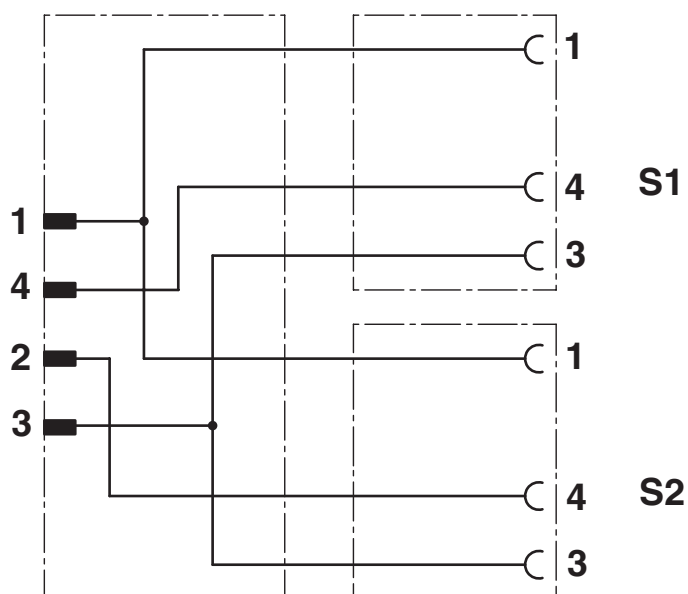
Contactbezetting van de M12-steker en de M8-bussen
