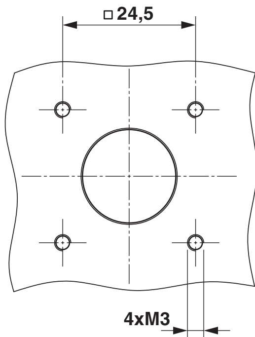
Maatschets
