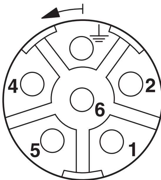
schematekening
