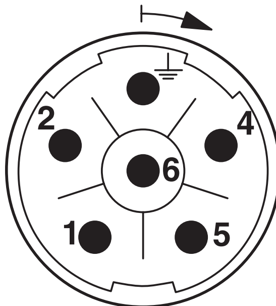
schematekening
