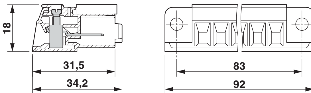
Maatschets
