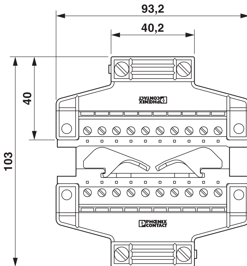
Maatschets
