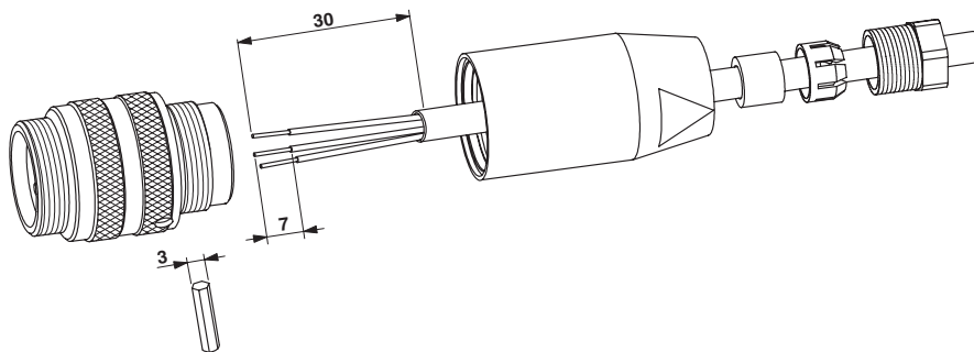
functietekening
