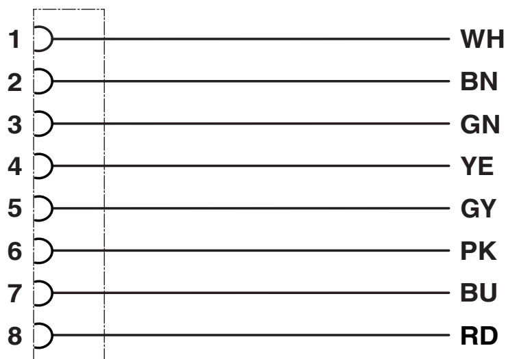
schakelschema
