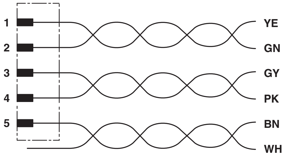
schakelschema
