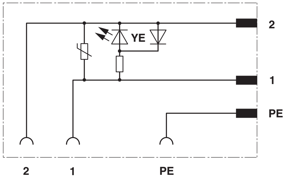
schakelschema
