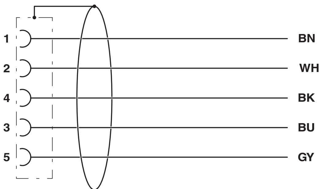
schakelschema
