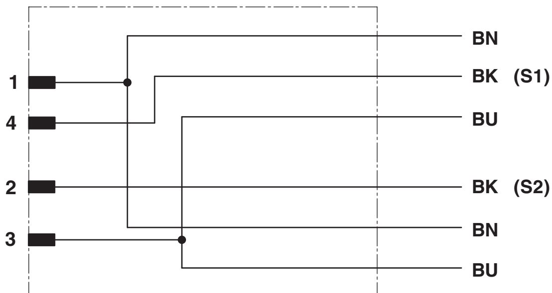
Contactbezetting van de M12-Y-stiftconnector
