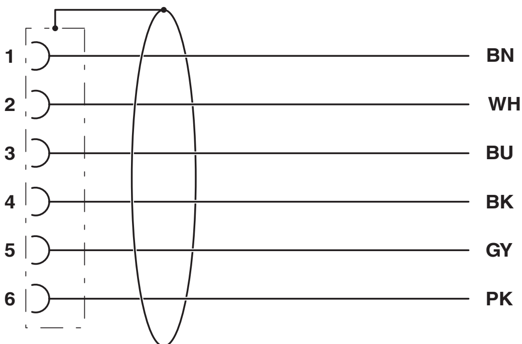
Contactbezetting van de M8-bus
