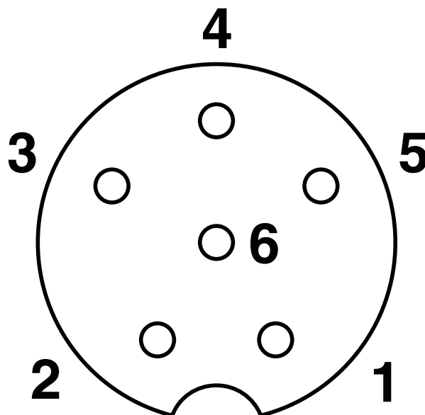
schematekening
