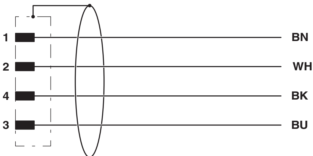
Contactbezetting van de M8-stekers/-bussen
