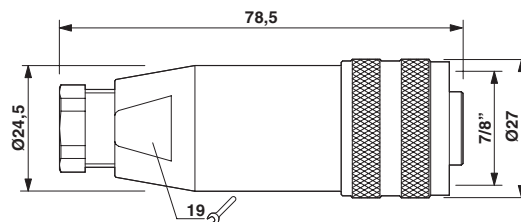
Maatschets
