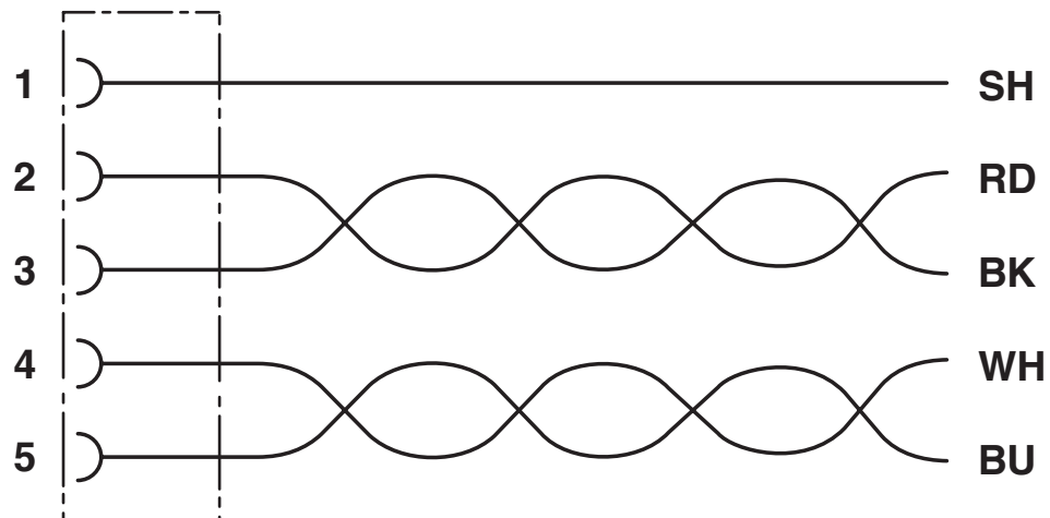
schakelschema
