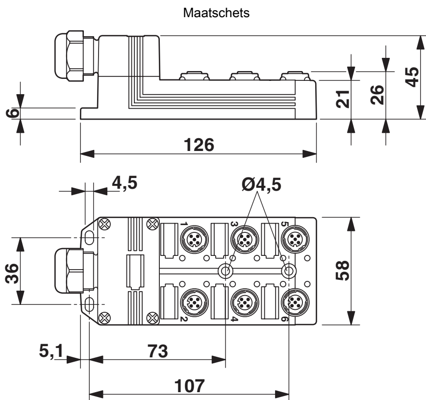
schematekening
