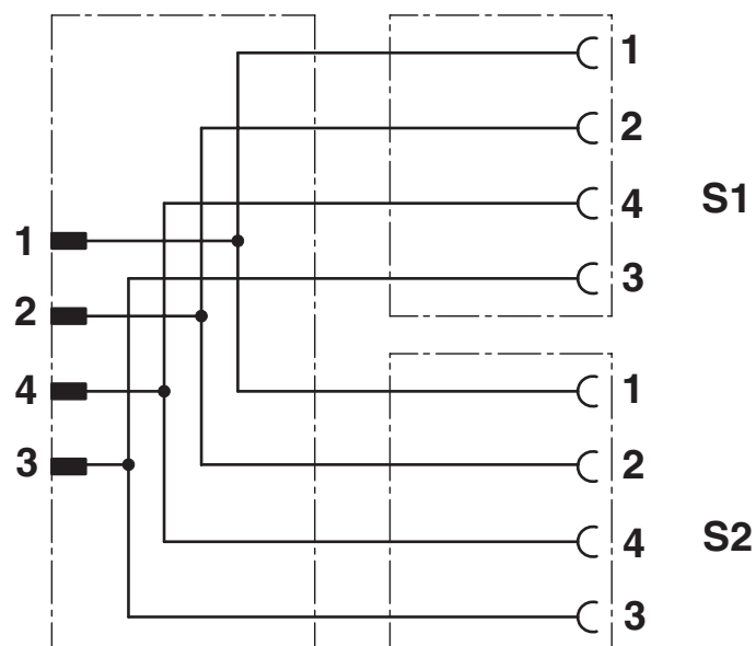
Contactbezetting van de M12-Y-steker en de M12-bussen
