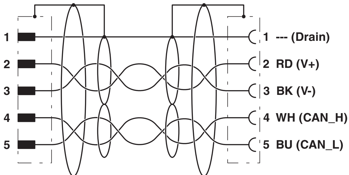
schakelschema
