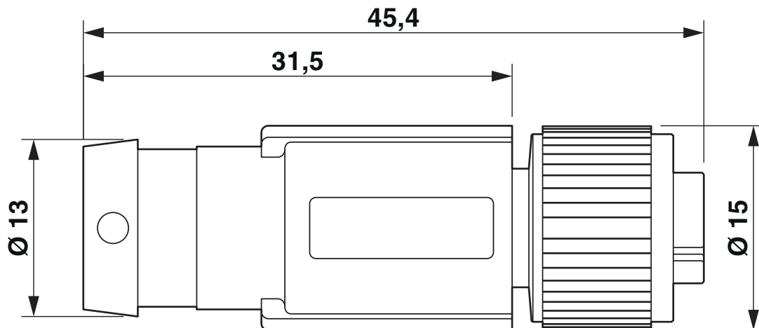
Maatschets
