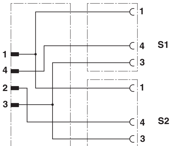
schakelschema
