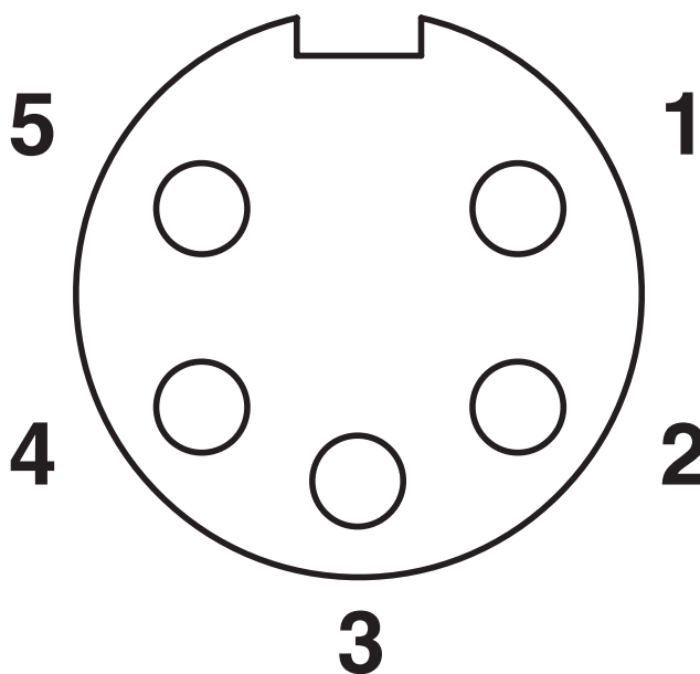
schematekening
