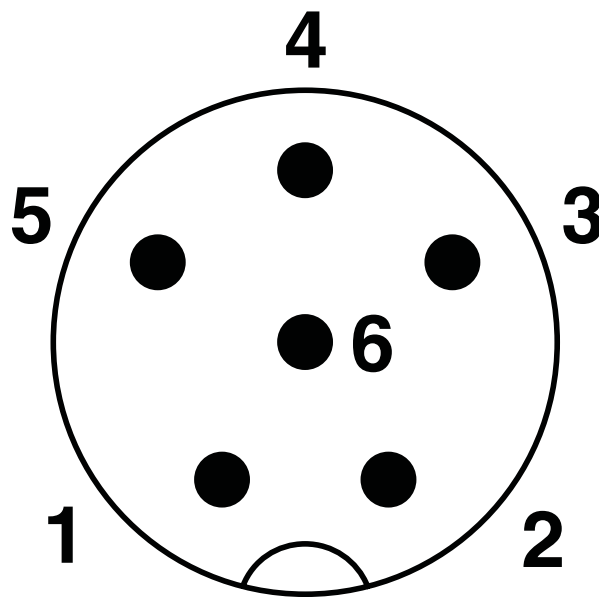
schematekening
