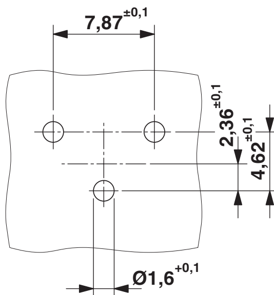
boorsjabloon/soldeerpadgeometrie
