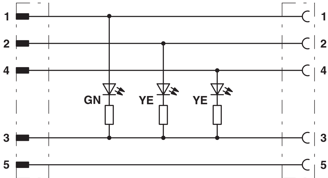
schakelschema
