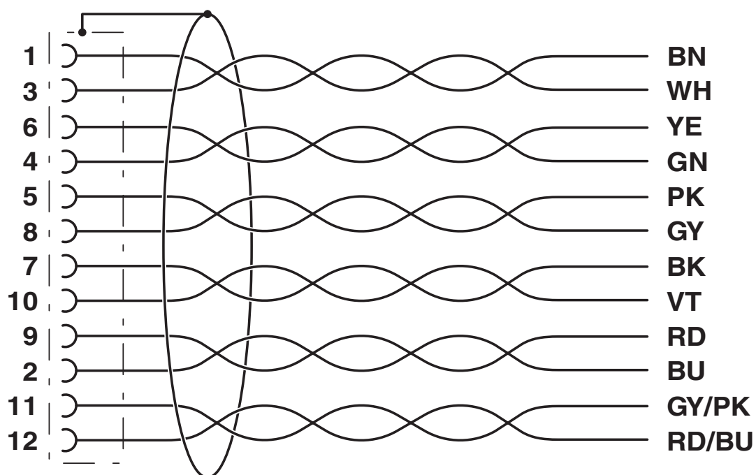
Contactbezetting van de M12-bus
