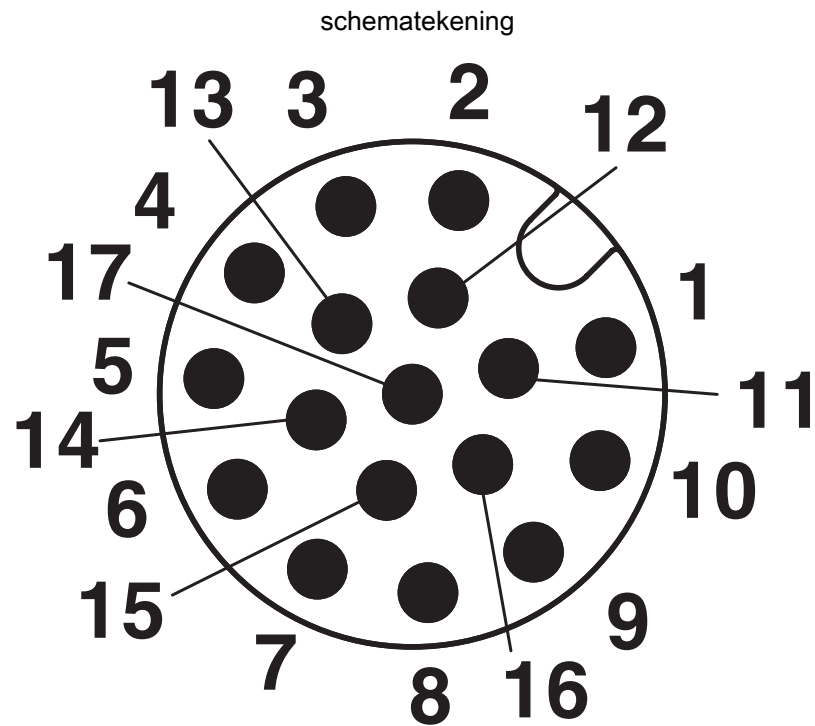
Poolschema steker M12, 17-polig, aanzicht stiftzijde
