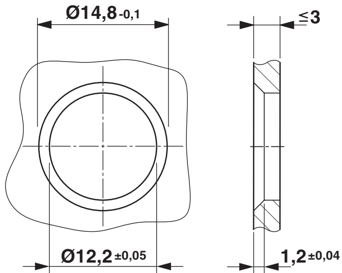
Maatschets
