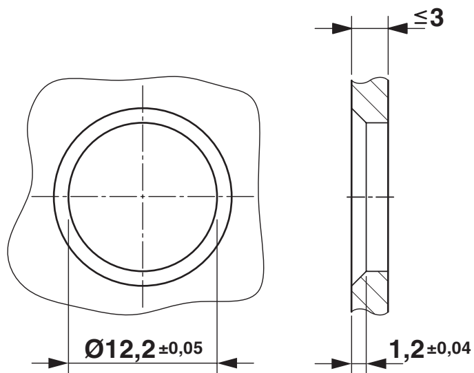
Maatschets
