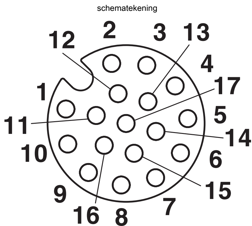
Poolschema bus M12, 17-polig, aanzicht buszijde
