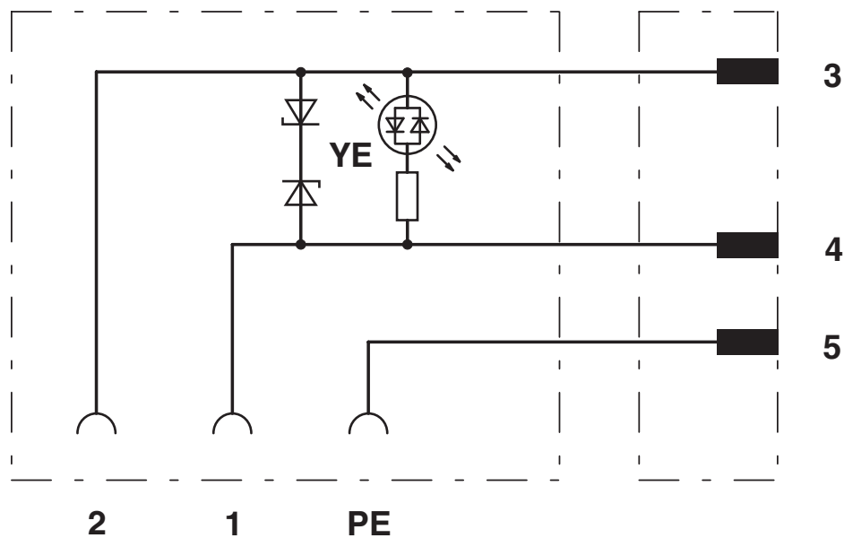
Contactbezetting van de M12-steker en de ventielsteker
