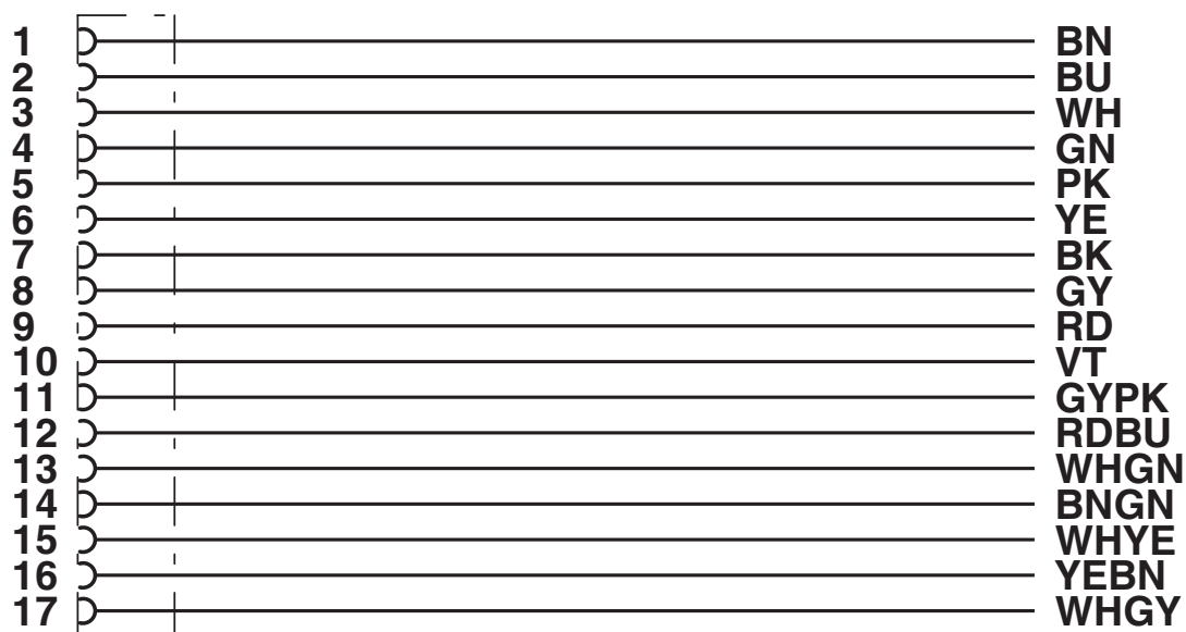
Contactbezetting van de M12-bus
