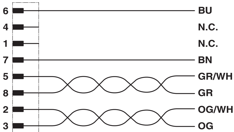
schakelschema
