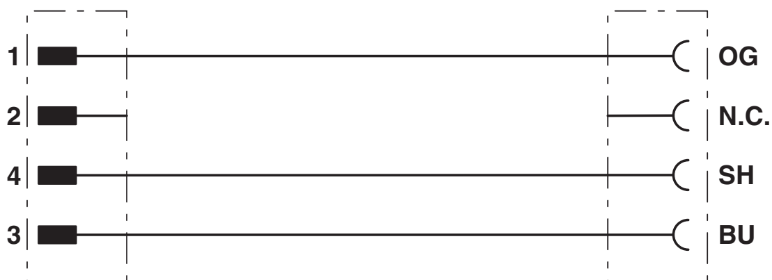
Contactbezetting van de M12-stiftconnector en de M12-busconnector
