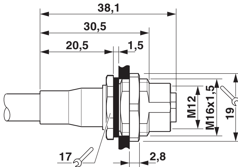
Maatschets
