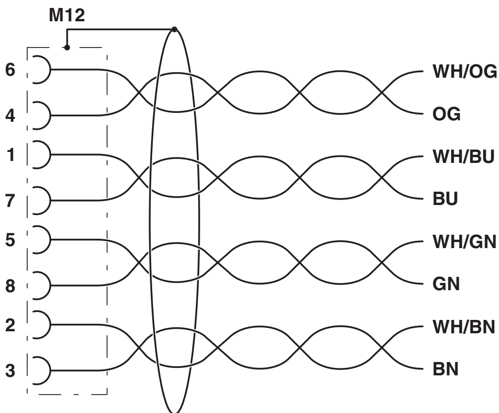
schakelschema
