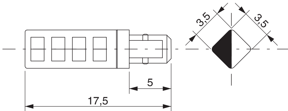
Maatschets
